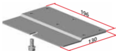
art. 2243 Staffa di fissaggio per tavoli scorrevoli Strap for sliding tables
