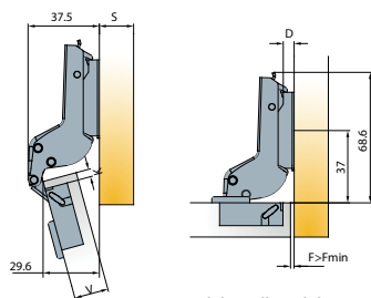
Risbe prikazujejo namestitev na D=2 mm montažno podlogo
