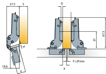
Risbe prikazujejo namestitev na D=0 mm montažno podlogo
