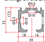
forature sull'art. 5801 drillings on the art. 5801
