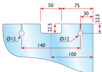
LAVORAZIONE VETRO WORKING GLASS
