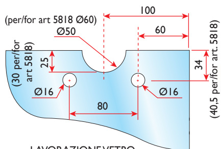
LAVORAZIONE VETRO WORKING GLASS
