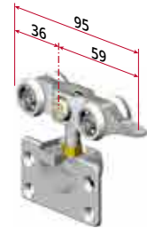
art. 2216/39 160* Carrello in acciaio regolabile completo di staffa art. 2239 Steel carriage adjustable with metal bracket art. 2239
