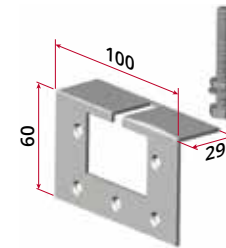
art. 2238 130* Staffa in acciaio con perno M8 Metal bracket with pin and nut M8
