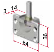
art. 2239 160* Staffa in metallo con incasso Ø35 mm completo di perno M8 Metal bracket Ø35 mm with threaded pin and nut M8
