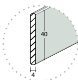
4 mm vetro temprato 4 mm tempered glass
