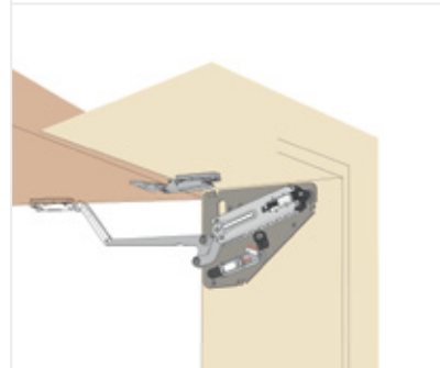
Regulacija mehkega zapiranja FLAP
