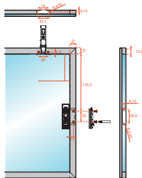
Načrt za pritrnitev pritrnilca na ALU ozek okvir
