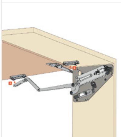
Pritrditev vrat na mehanizem FLAP
