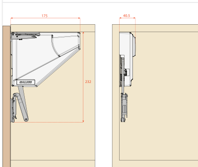
Dimenzije mehanizma FLAP
