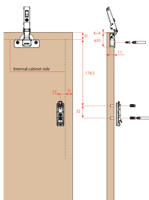
Načrt za pritrnitev pritrnilca na lesena vrata
