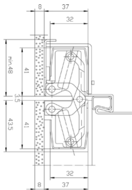
Montaža na jeklenih podbojih
