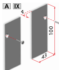
Art. 5830 Za art. 5801-5810
