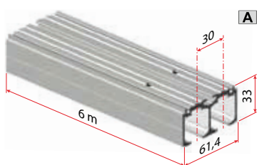
Art. 5832 40÷160
