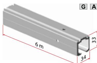
Art. 5801 40÷160 Kg
