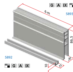
Art. 5893 - art. 5892 Za art. 5801-5832-5833-5809
