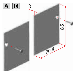
Art. 5839/2 Za art. 5832-5809
