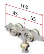
Art. 2434 130Kg
