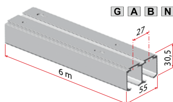
Art. 2242 40÷160 Kg
