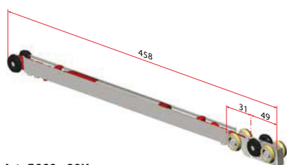
Art. 5669 80Kg Za art. 5666
