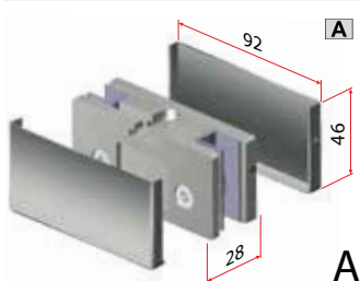
Art. 3401 130Kg
