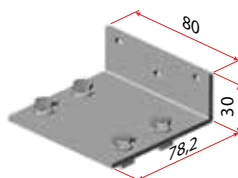
Art. 5823 Za art. 5833-5832-5893
