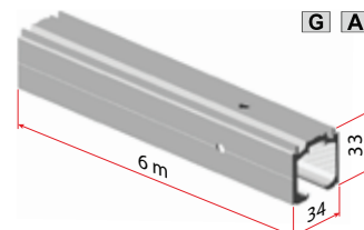
Art. 5801 40÷160 Kg
