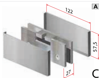
Art. 5818/A 150Kg
