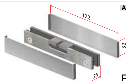
Art. 5814/A 130Kg
