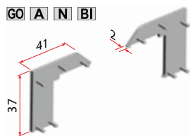
Art. 4211 Za art. 4201-4204/41-2201
