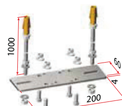
Art. 245 Za art. 2422/41 - 2201
