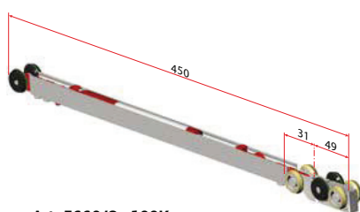
Art. 5669/S 100Kg Za art. 5666/S
