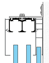
2A-PV Stenska montaža s fiksnim steklenim panelom
