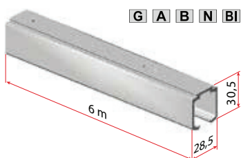
Art. 2201 40÷160 Kg
