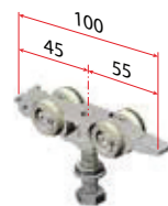
Art. 2434/35 130Kg
