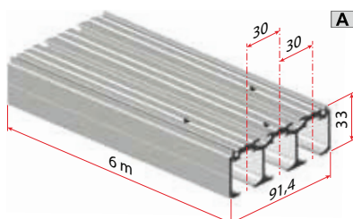
Art. 5833 40÷160 Kg
