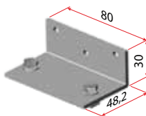
Art. 5822 Za art. 5832
