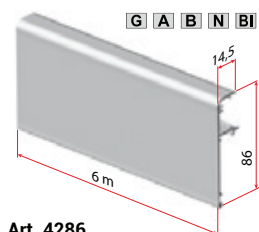
Art. 4286 Za art. 2201-2242
