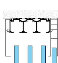
3A-S Stropna montaža s fiksnim steklenim panelom
