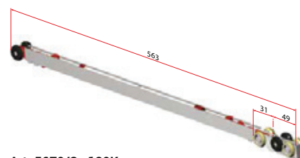
Art. 5679/S 130Kg Za art. 5666
