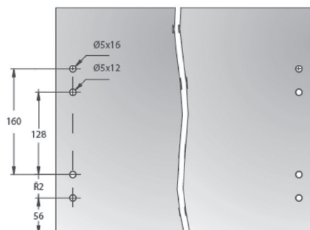
Mere za pritrditev prekucnika na ličnico
