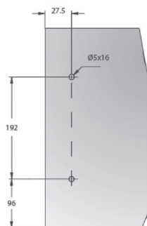
Mere za pritrditev na stranico elementa
